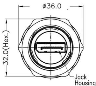
Conn.1
