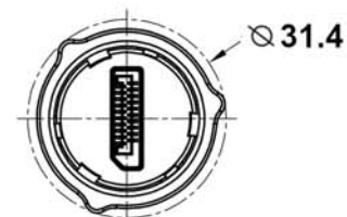
Conn.1
