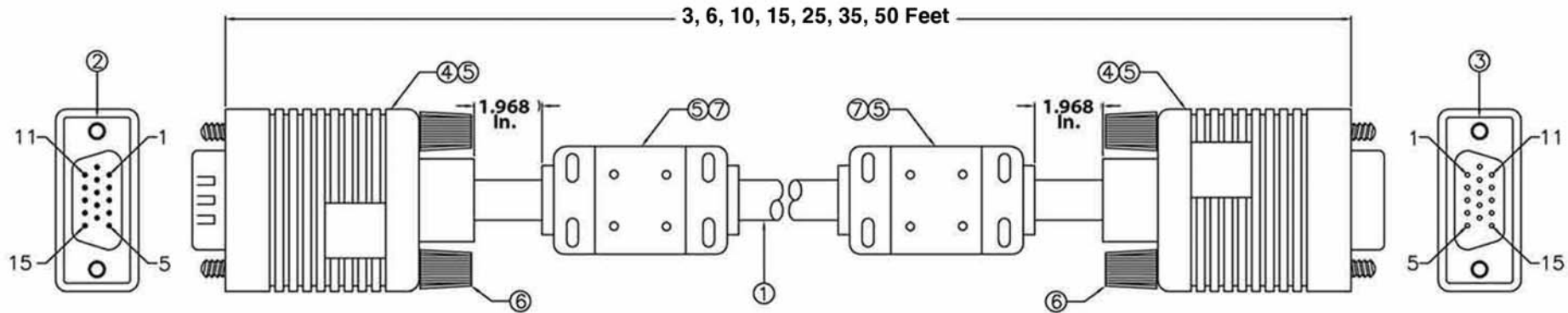
Conn.1 HDB15P/M
